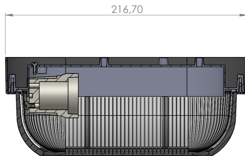
SEÇÃO A-A
